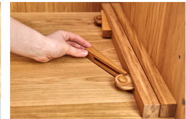
6. Deckplatte, Bodenplatte, Seitenwand und Innenrahmen miteinander verbinden: zuerst Holzdübel durch die Lasche stecken, dann Spannkeil auf die Lasche stecken und gefühlvoll „auf Zug“ festklopfen.
